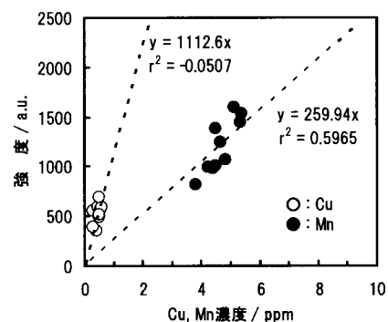
図3 ホタテガイ貝殻製蛍光体の個体差によるCu濃度と490nm発光帯強度、およびMn濃度と580nm発光帯強度との関係
