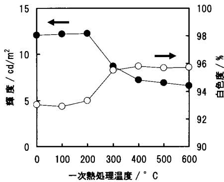
図7 一次熱処理温度によるホタテガイ貝殻製蛍光体の輝度および白色度
